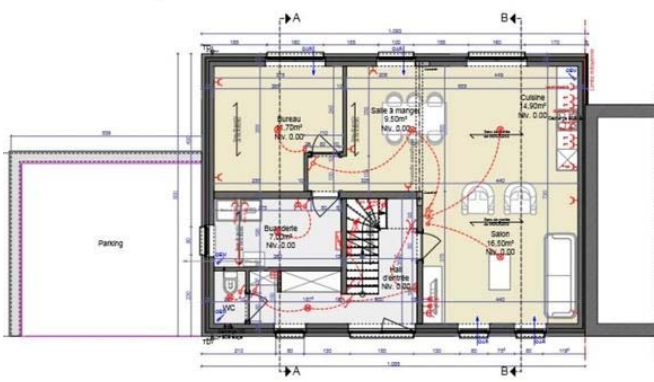
Intérieur DM1 - Couverture d'Alimentation Régulée Intérieur DM1 - Couverture d'Évacuation Mécanique
